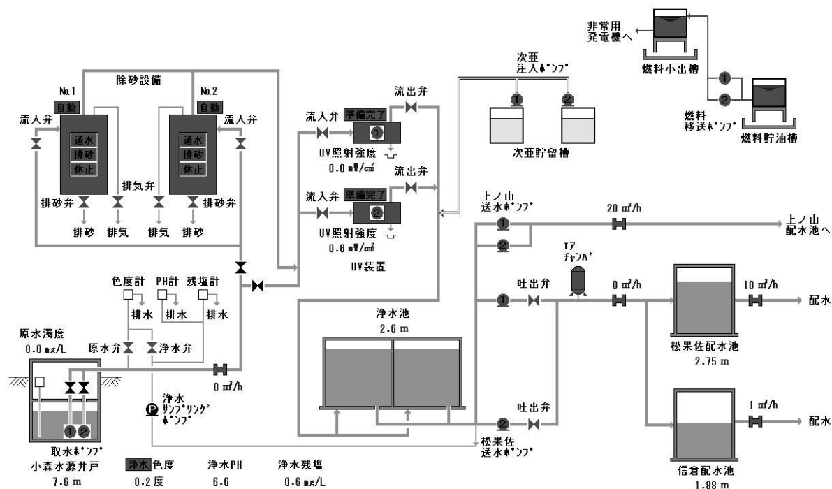
図. 小森浄水場フローチャート
