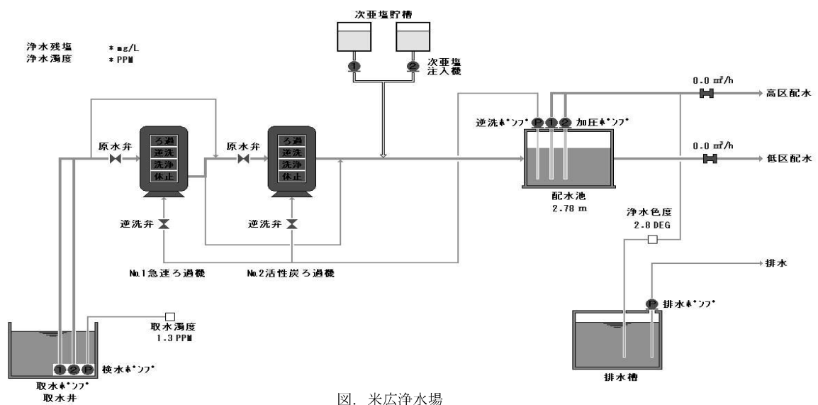
図. 米広浄水場
