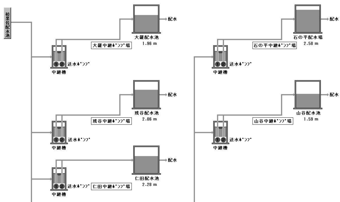
図. 入谷系中継ポンプ場・配水池
