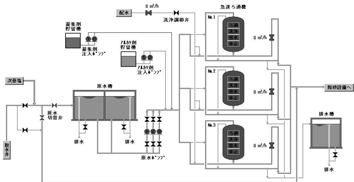
図. 新戸倉浄水場（濁度 2 超時）
