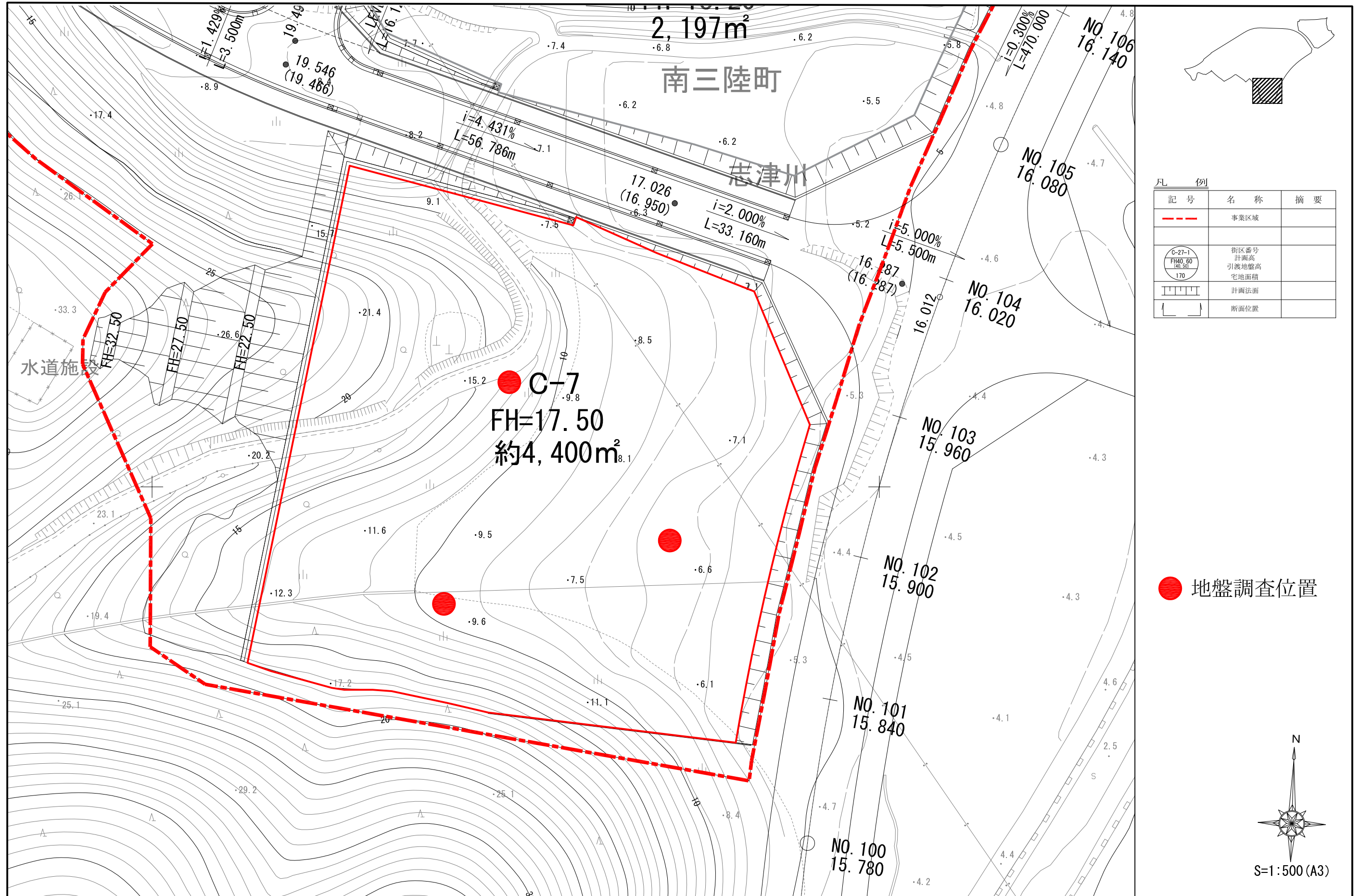
図3 地盤調査位置図
