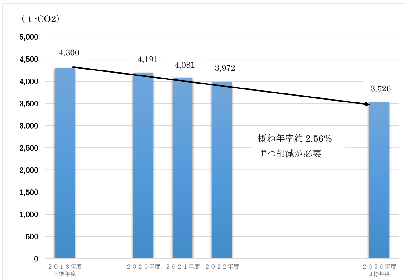
図5 温室効果ガスの削減目標
