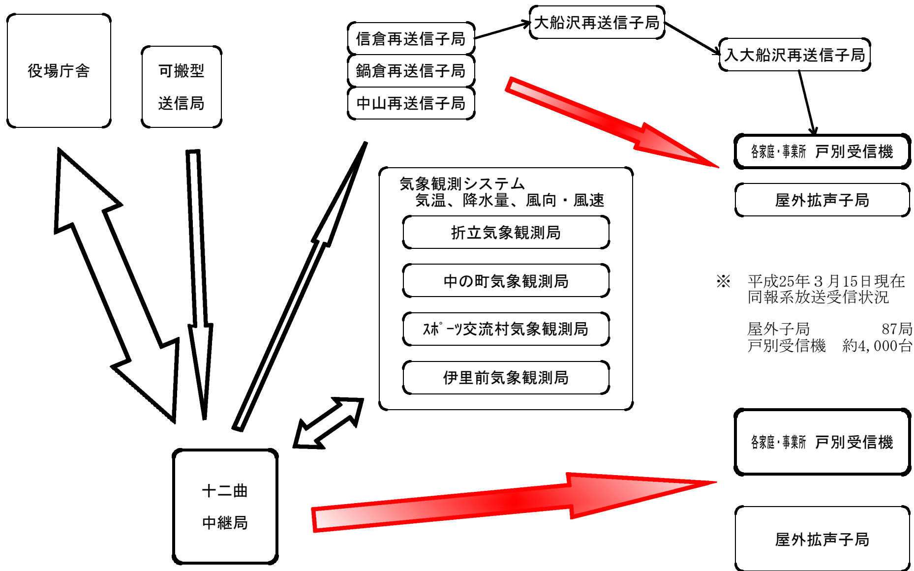
南三陸町防災行政無線（同報系）通信体系図
