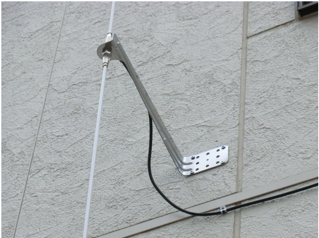
ダイポールアンテナ設置の例（役場庁舎壁面）
