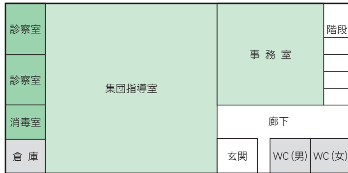
志津川保健センター 平面図
